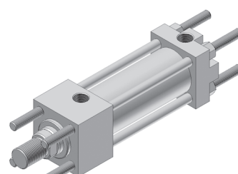
Montagem por Tirante Tipo Extensão Dianteiro e Traseiro (pág. 11)
