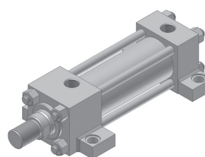
Montagem Sapatas Laterais na Base (pág. 16)
