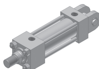
Montagem Aleta Dupla Traseira (pág. 13)
