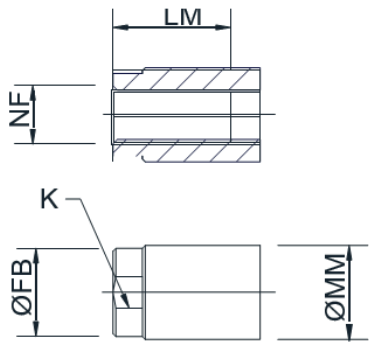
ROSCA INTERNA
