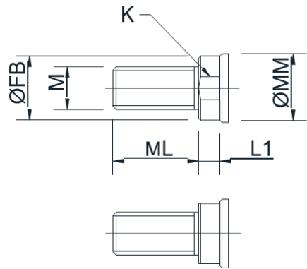
ROSCA EXTERNA
