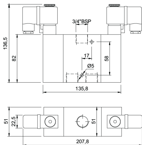
Solenoide Diferencial 3 Vias
