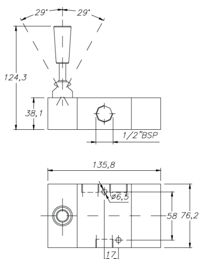
Duplo Piloto 3 Vias - 3 posições
