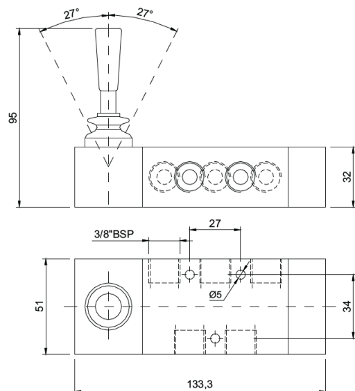
Alavanca Diferencial 5 Vias - 3 posições
