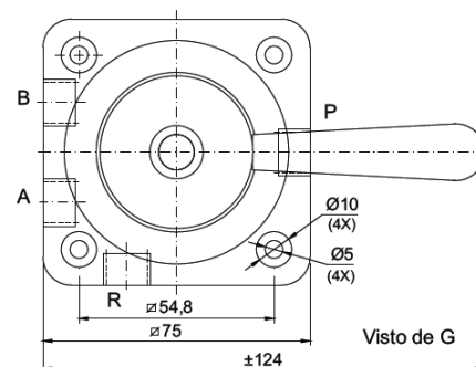
Saída lateral
