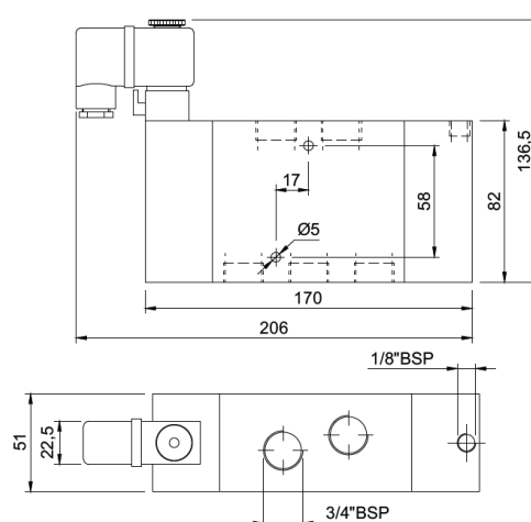
Solenoide Piloto 5 Vias
