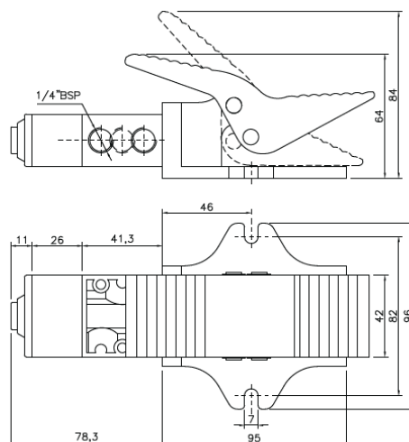
Pedal Mola 3 Vias - 3 posições
