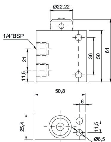
Piloto Mola 3 Vías
