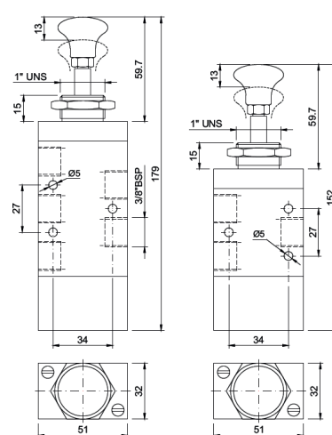
Duplo Piloto 5 e 3 vias
