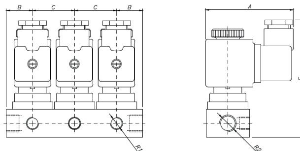
Bloco com bobina Grande***
