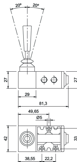
Alavanca Trava 3 Vias - 3 posições
