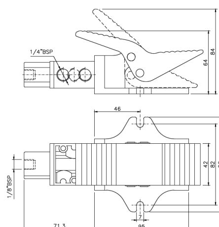
Pedal Diferencial 3 vias
