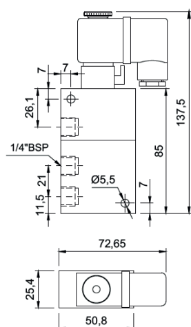
Solenoide Mola 3 Vías
