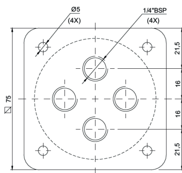
Saída na base
