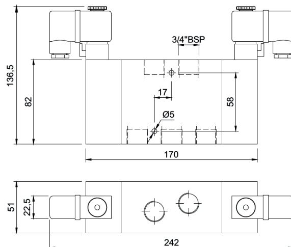
Solenoide Diferencial 5 Vias
