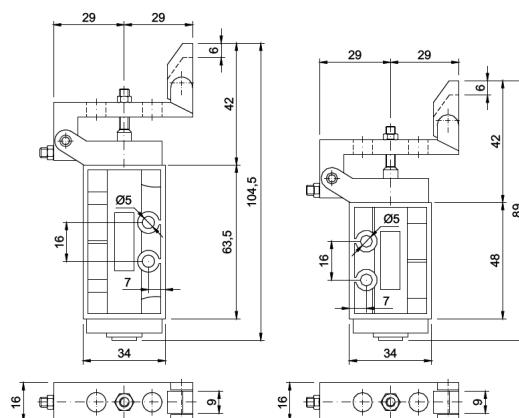
Gatilho Mola 5 e 3 vias
