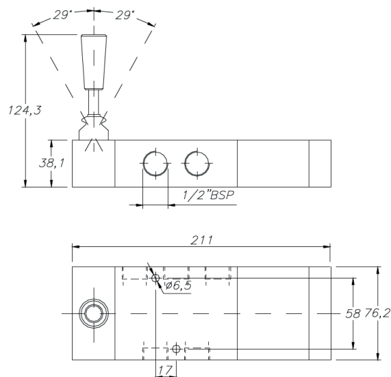
Alavanca Mola 5 Vias - 3 posições
