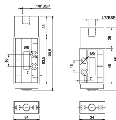
Piloto Mola 5 e 3 vias
