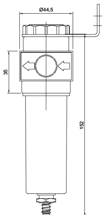
Filtro de Ar - FT
