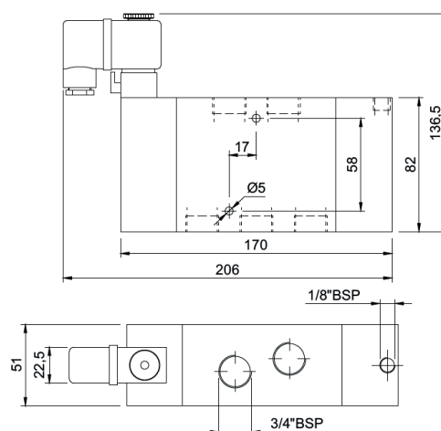
Solenoide Piloto 5 Vias
