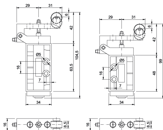
Roleta Mola 5 e 3 vias
