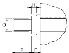
Detalhe da haste com rosca externa
