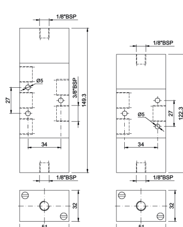
Alavanca Trava/Diferencial 3 vias
