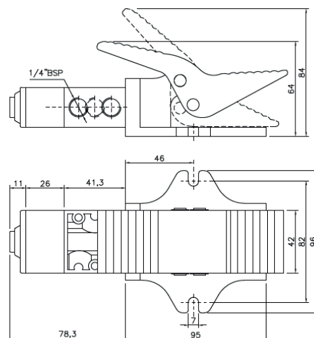
Pedal Mola 3 Vias - 3 posições
