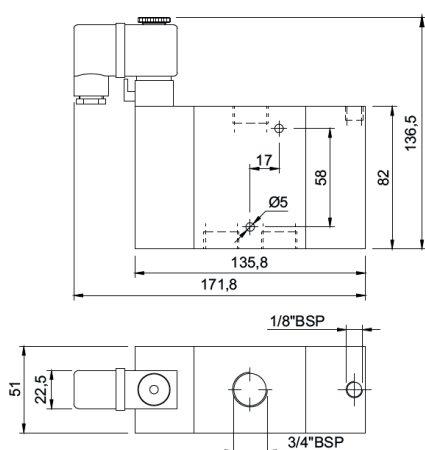
Solenoide Piloto 3 Vias
