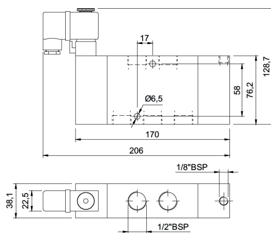
Piloto Diferencial 5 Vias
