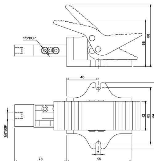
Pedal Piloto 3 vias
