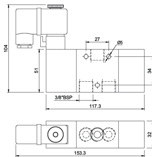
Solenoide Diferencial 3 vias
