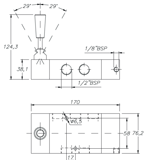
Alavanca Diferencial 5 Vias
