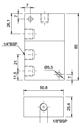
Solenoide Mola 3 Vías
