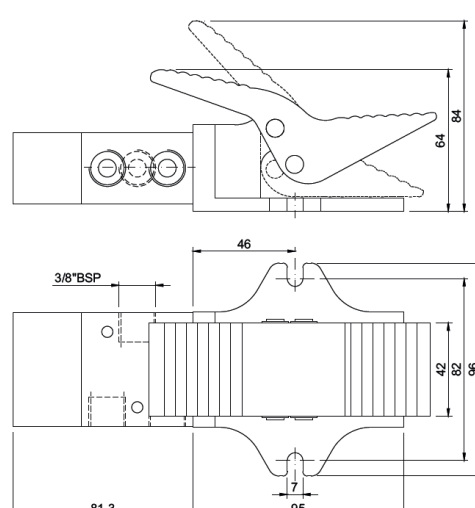
Pedal Diferencial 3 vias
