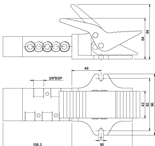
Pedal Diferencial 5 vias
