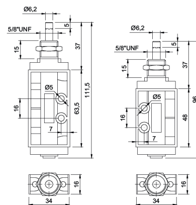
Pino Mola 5 e 3 vias
