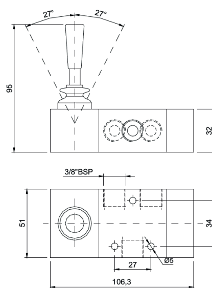
Alavanca Diferencial 3 Vias - 3 posições
