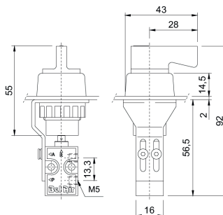
8. Seletor Longo / Trava
